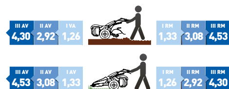
SNELHEIDSGRAFIEK IN KM/H MET WIELEN 5.0-10
